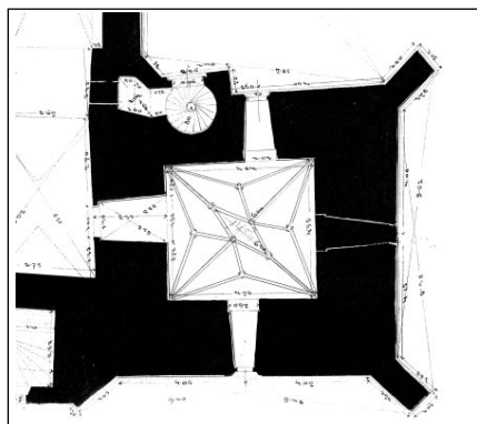
Obr. 6. Půdorys přízemí (kaple Božího hrobu s hvězdicovou klenbou) věže chrámu sv. Petra a Pavla (Stavební archiv Městského úřadu Mělník)
