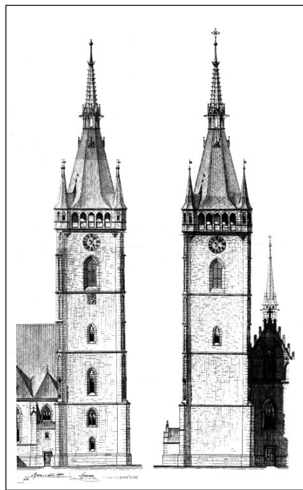
Obr. 5. Nerealizovaná rekonstrukce věže chrámu sv. Petra a Pavla, severní (a) a západní (b) průčelí, návrh: Josef Mockera, 1894 (Stavební archiv Městského úřadu Mělník)
