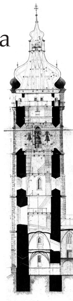
Řez věží kostela, ale kterého je její výška včetně kříže 65 m (Stavební archiv Městského úřadu Mělník)
