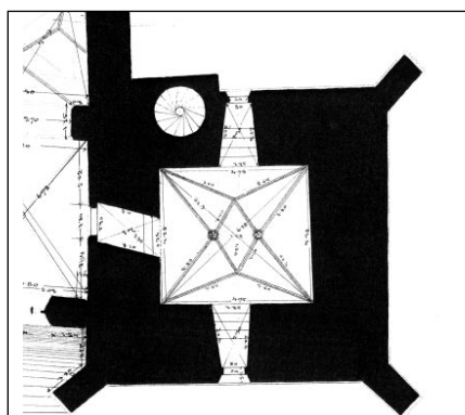
Obr. 7. Půdorys věže chrámu sv. Petra a Pavla ve výšce choru (komoře - trezor s hvězdicovou klenbou) (Stavební archiv Městského úřadu Mělník)
